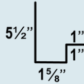
Door Jamb
