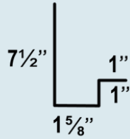
Door Jamb
